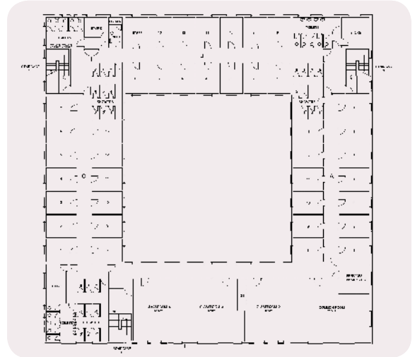
الطابق الثاني
